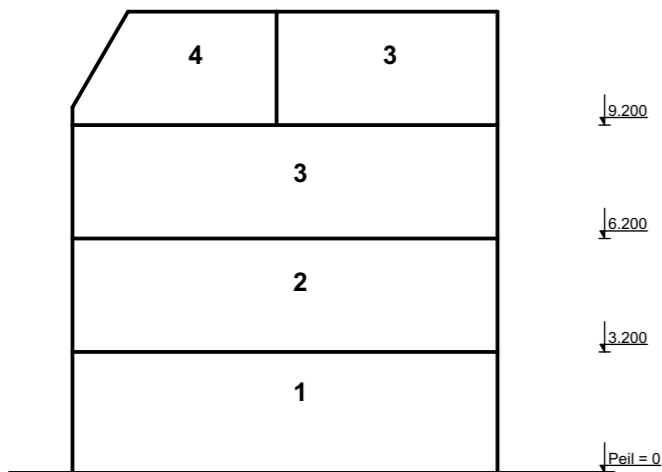
Doorsnede A-A schaal 1:200
